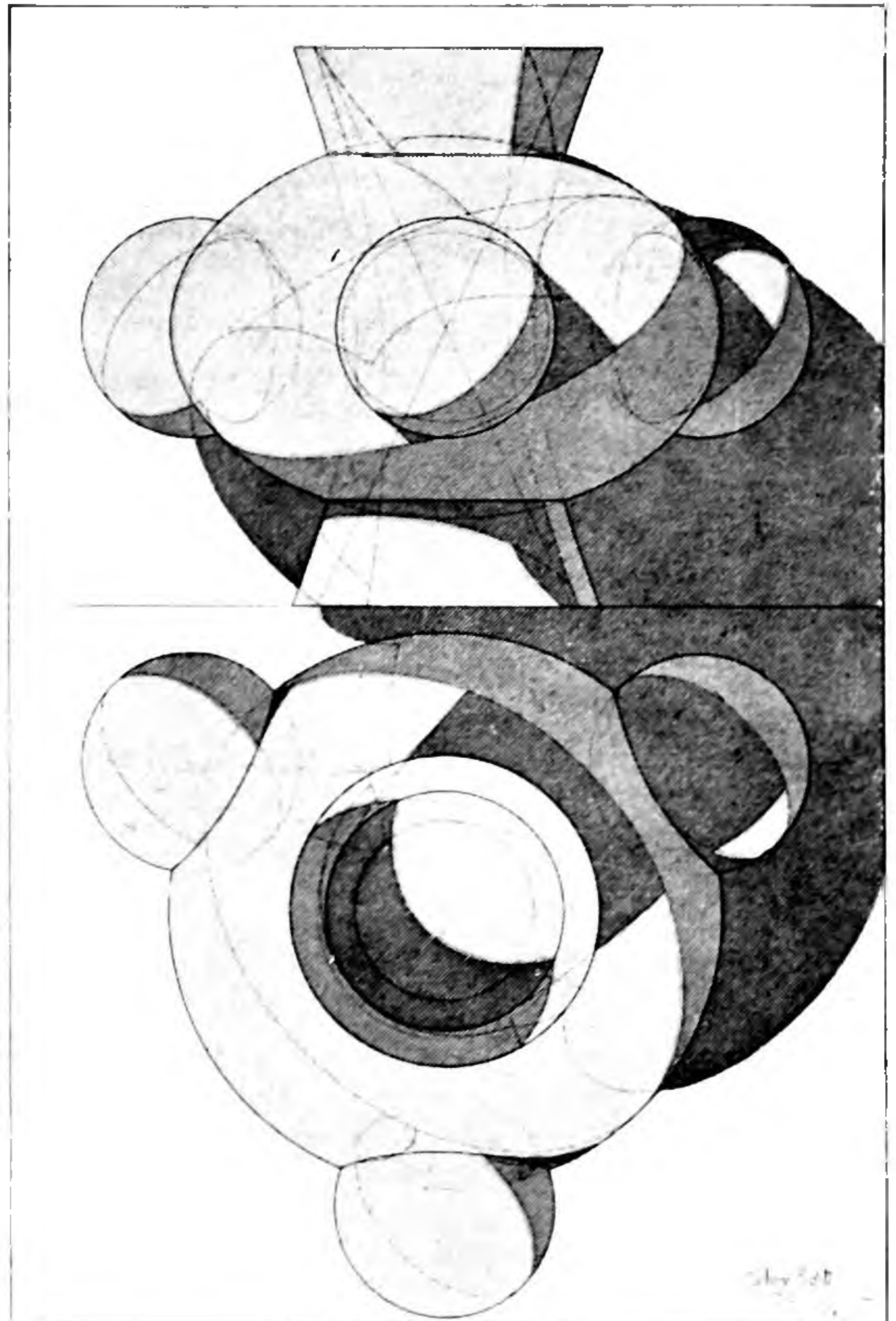
Durchdringungs- und Beleuchtungsaufgaben von Rotationsflächen in orthogonalen Projectionen. Professor: G. Kovách.
