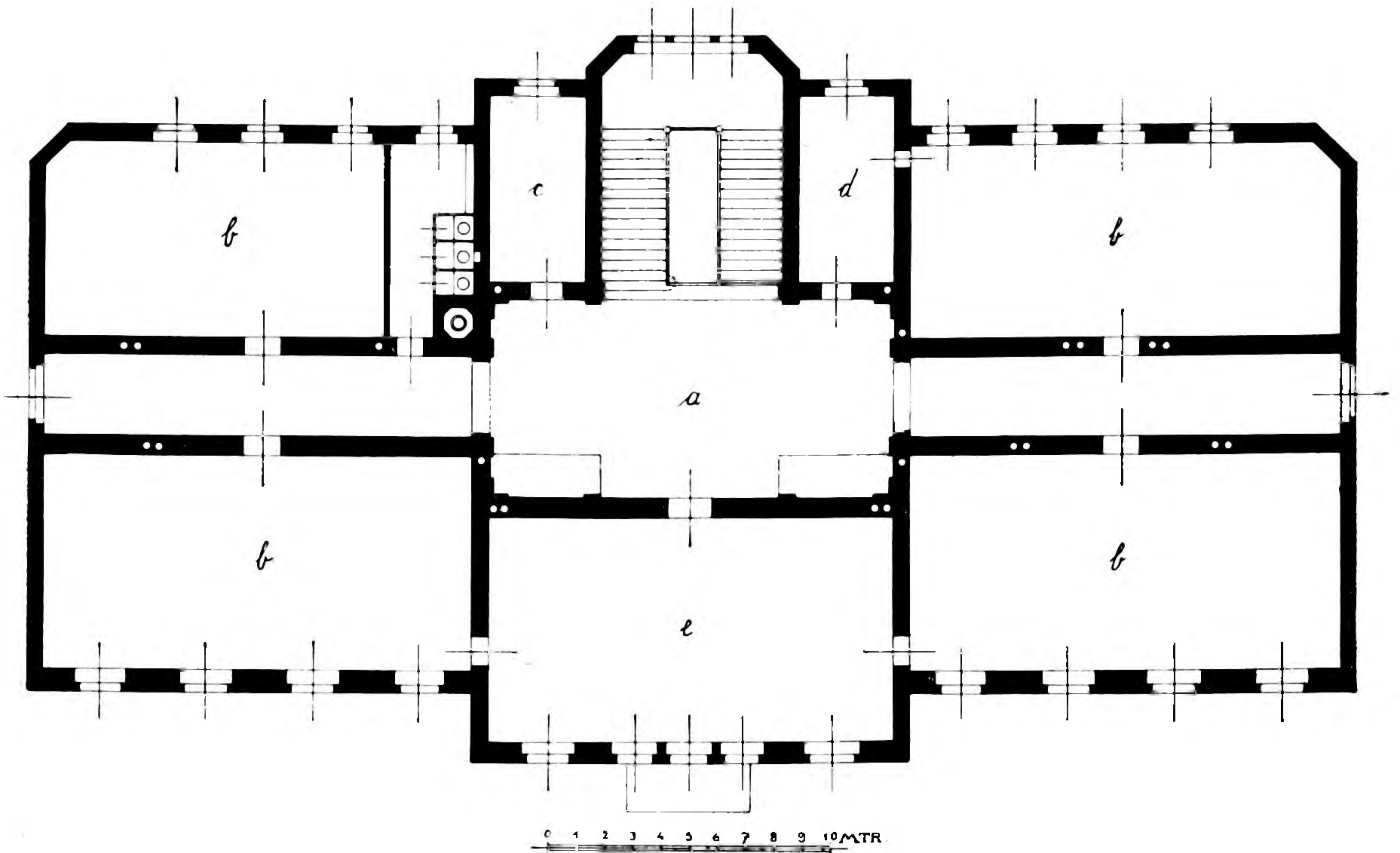
a Halle; b Bibliotheksäle; c , d Zimmer des Bibliothekars und des Aufsehers; e Lesesaal.
