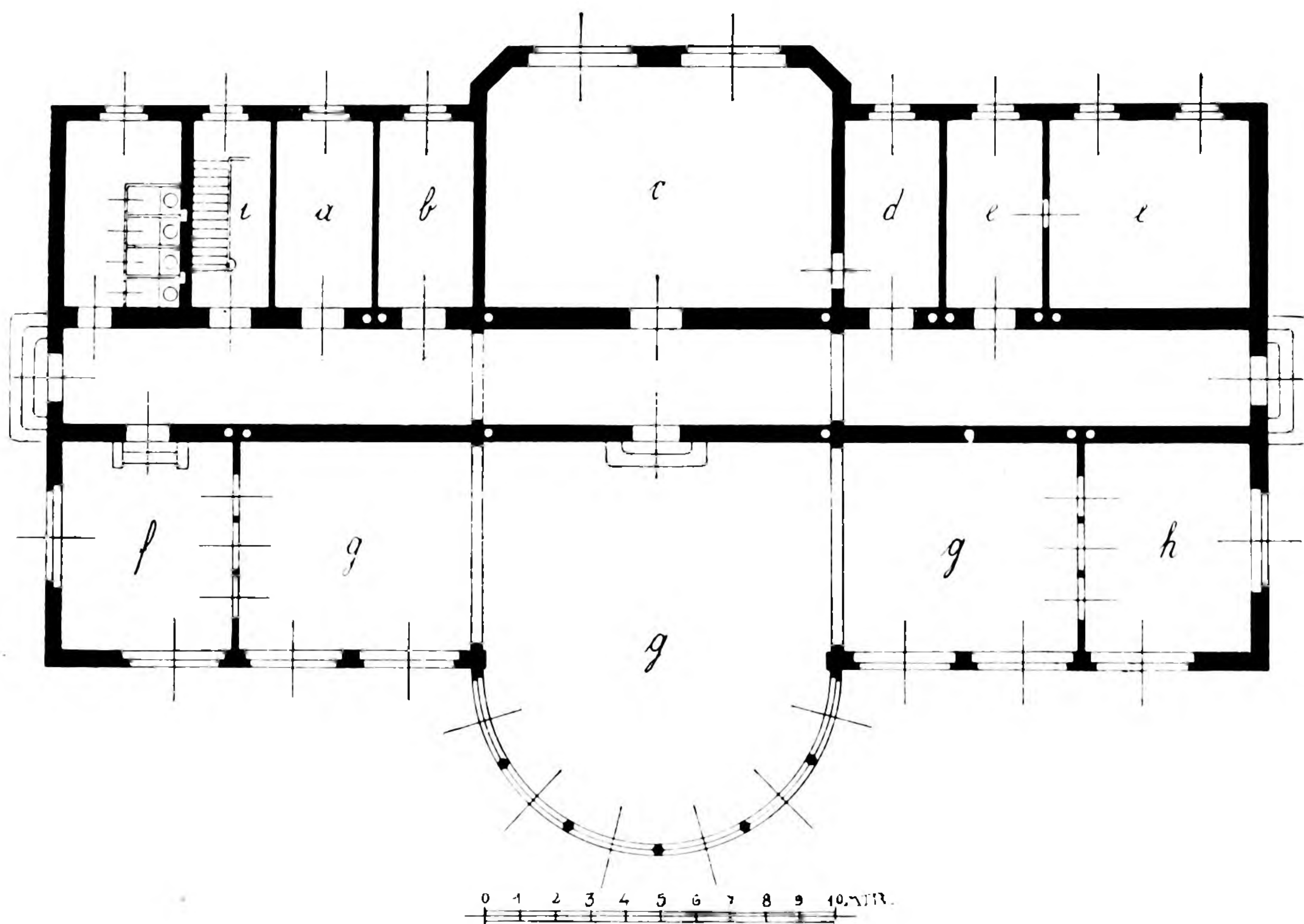
a Requisitenstube; b Dienerstube; c Zeichensaal; d Professoren-Zimmer; e Schuldiener-Wohnung; Raum für lebende Vögel; g h Gewächs- und Blumenhalle; i Bodenstiege.
