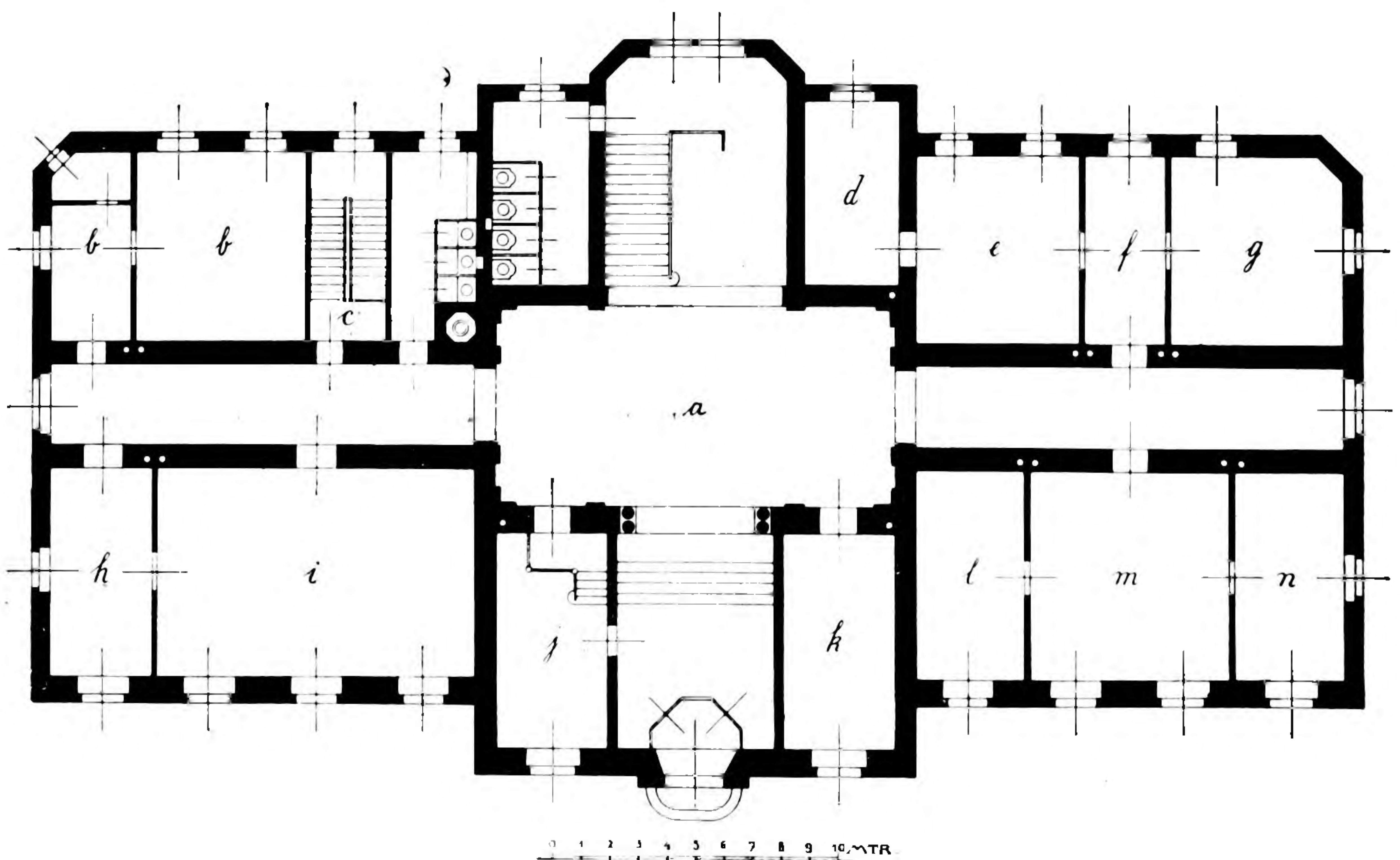
a Vorhalle; b Portierwohnung; c Kellerstiege; d , n , h Archive; e und g Empfangssäle der Direktoren; k und i Vereinslokale der Studierenden; j Portierloge; l , m und n Direktions-Bureaux.
