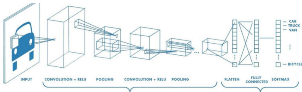
102. kép Convolutional Neural Networks (CNN)
