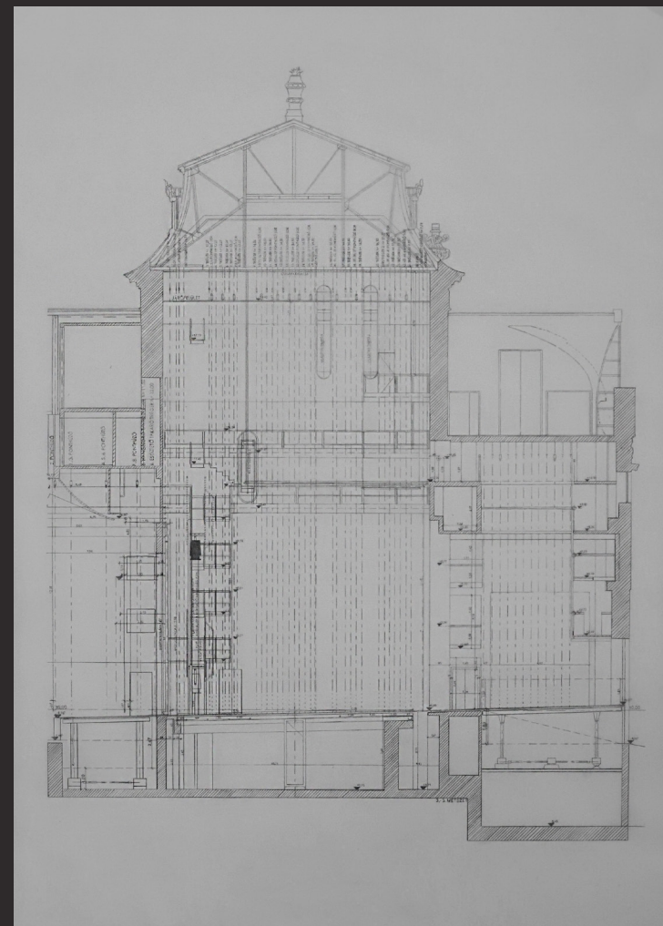
Metszet
